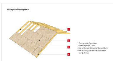
Verlegeanleitung für den Einsatz der SWISS KRONO OSB/3 bright im Dachbereich (Bildnachweis: INTERSPAN Faipari Kft.)
