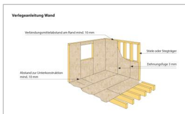
Verlegeanleitung für den Einsatz der SWISS KRONO OSB/3 bright im Wandbereich (Bildnachweis: INTERSPAN Faipari Kft.)
