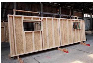
Vorfertigung von Wandelementen aus SWISS KRONO OSB/3 bright (Bildnachweis: SWISS KRONO)
